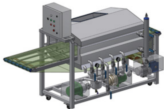
WASHING CONVEYOR SYSTEM Рыбомоечная машина конвейерного типа
