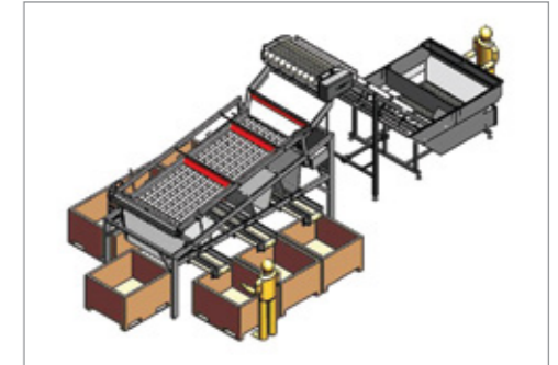
FISH GRADING LINE Сортировочная линия
